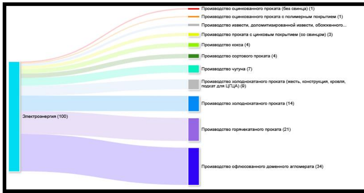
Рисунок 1.2. Потребление электроэнергии по технологиям производства
