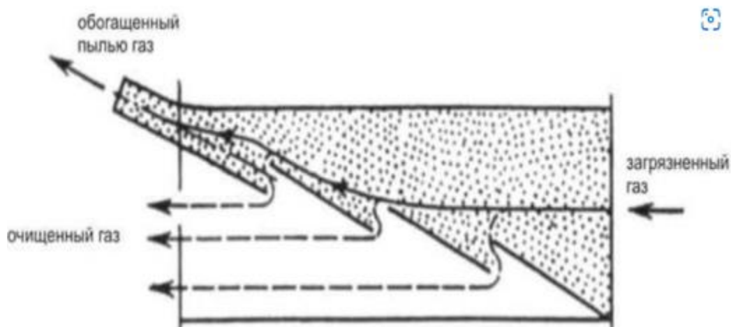
Рисунок .10. Жалюзийный пылеотделитель
