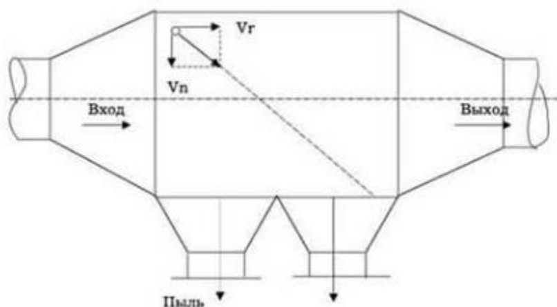
Рисунок 5.9. Схема горизонтальной осадительной системы
