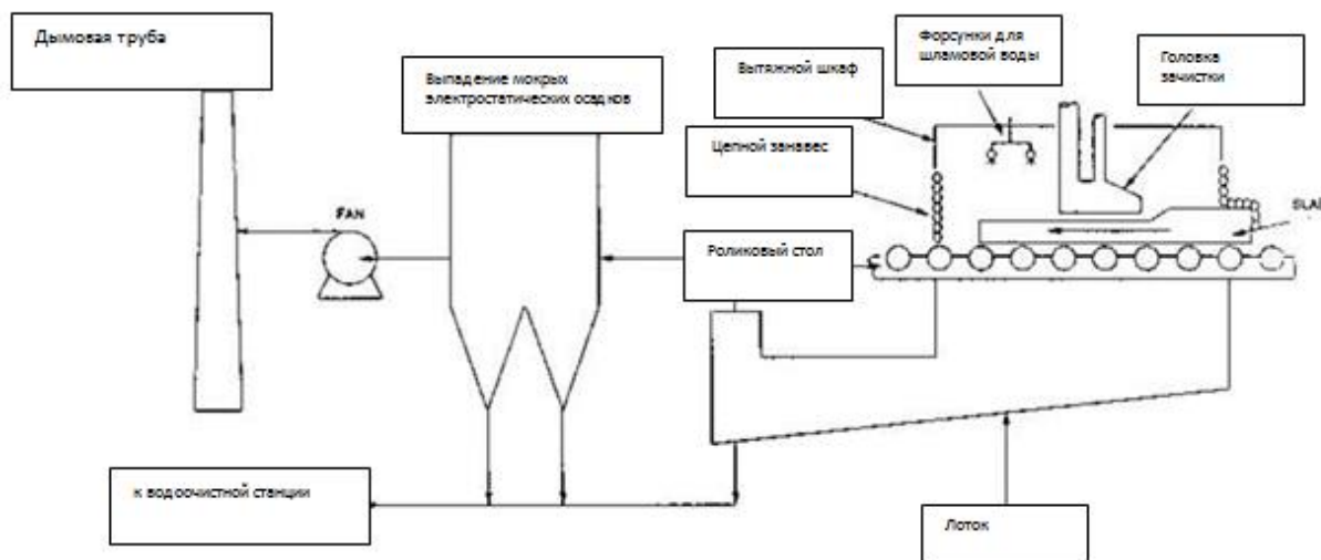
Рисунок 5.3. Технологическая схема предотвращения с загрязнением при закрытой зачистке (пример с влажным электрофильтром)
