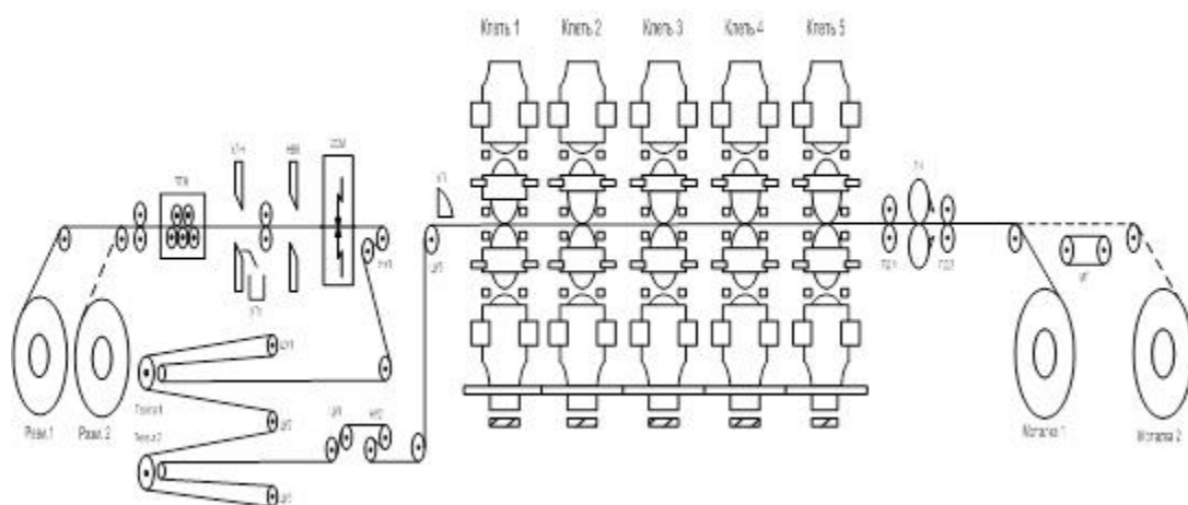
Рисунок 3.7. Технологическая схема непрерывного 5 клетьевого стана 1700 холодной прокатки рулонов
