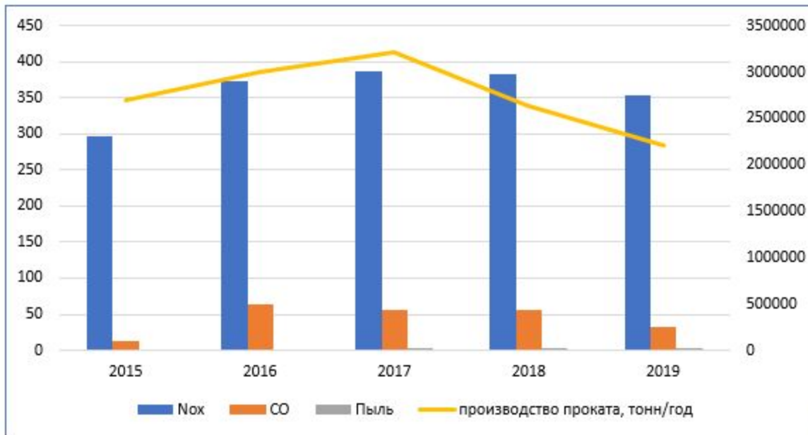
Рис.1.5. Выбросы и удельные показатели ЗВ за 2015–2019 гг. (от производства горячекатаного плоского проката).
