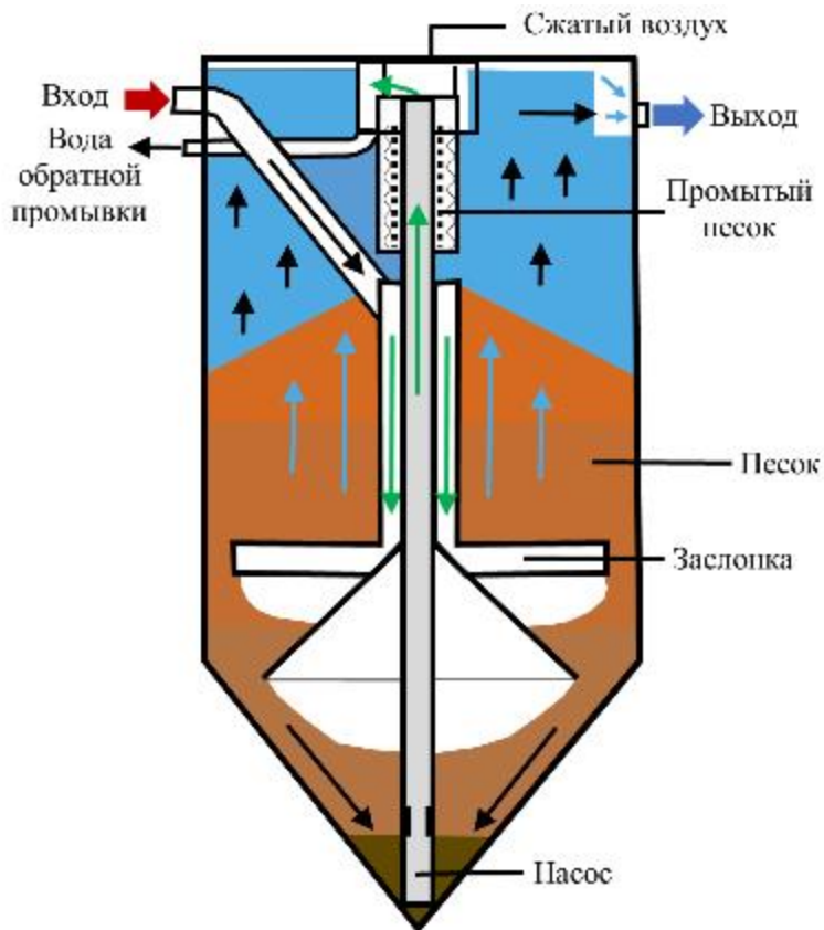
Рисунок .25. Схема песчаного фильтра
