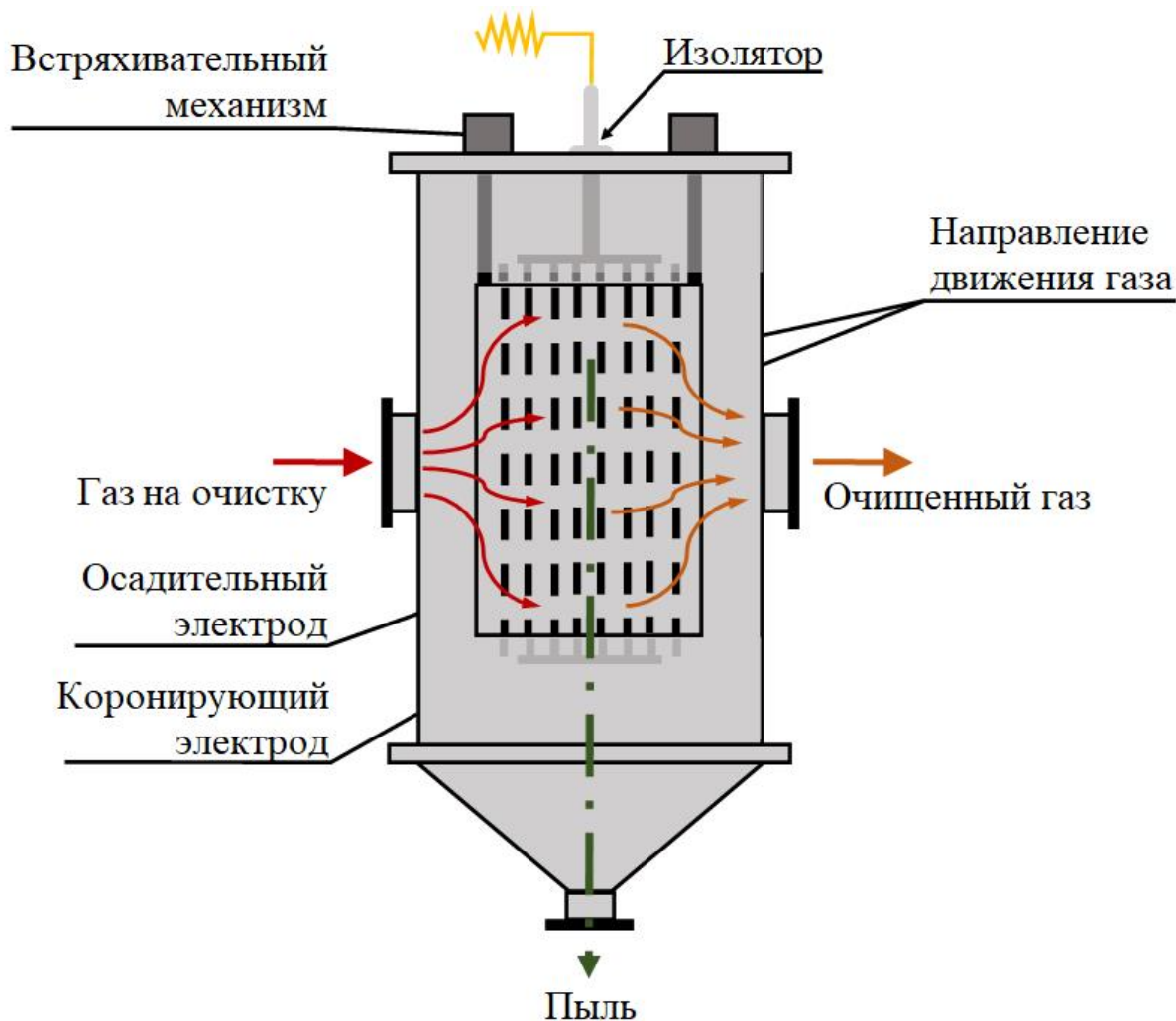
Рисунок .12.Схема устройства электрофильтра (показаны только две зоны)
