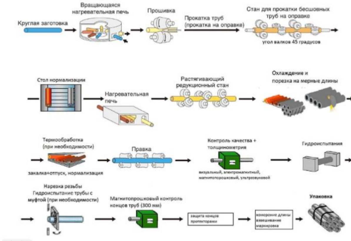
Рисунок 3.16. Схема производства обсадных и насосно-компрессорных труб
