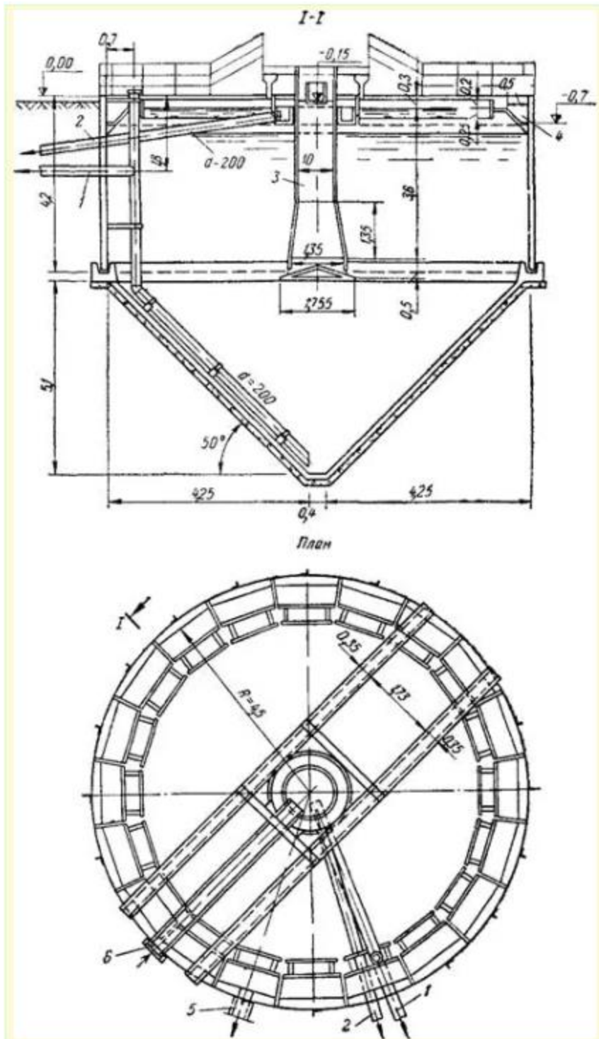
Рисунок .24. Конструкция вертикального отстойника
