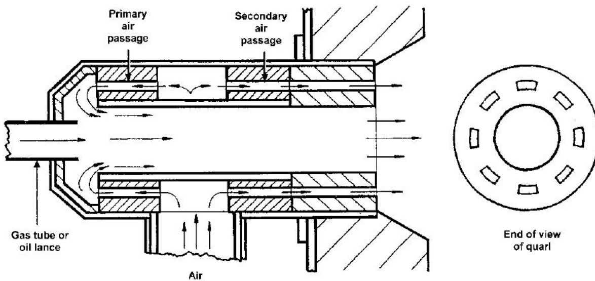
Рисунок 5.17. Схематический пример горелки с низким содержанием \text{NO}_x , работающей на воздухе
