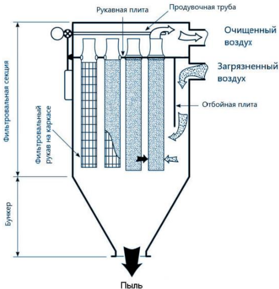
Рисунок 5.13. Конструкция рукавного фильтра
