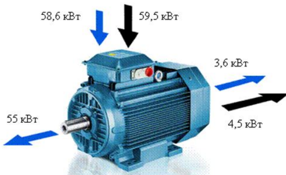
Рисунок .5. Сравнение обычного электродвигателя с энергоэффективным Достигнутые экологические выгоды
