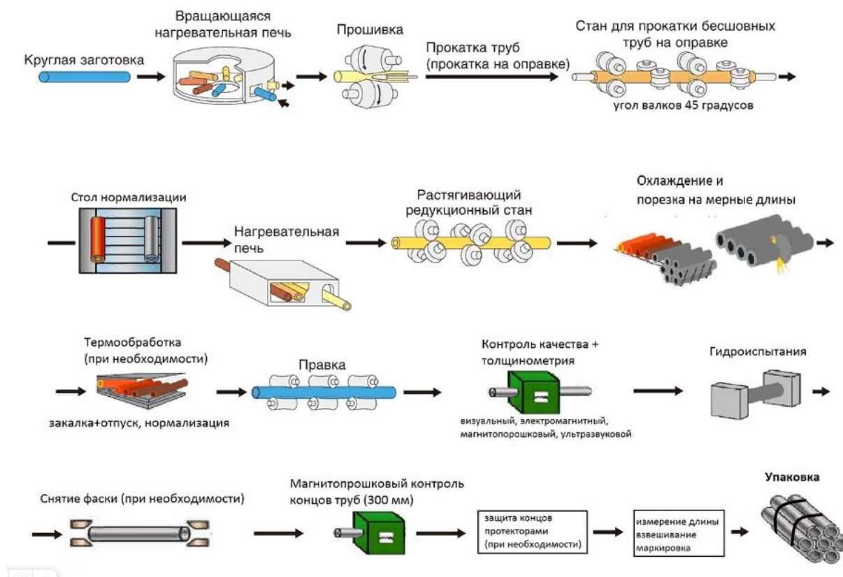
Рисунок 3.15. Схема производства нефтегазопроводных труб
