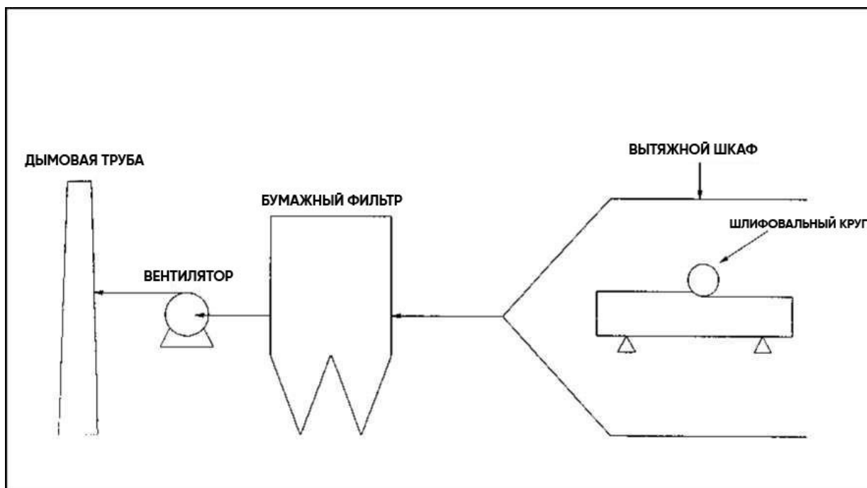
Рисунок 5.4. Технологическая схема с предотвращением загрязнением в процессе зачистки
