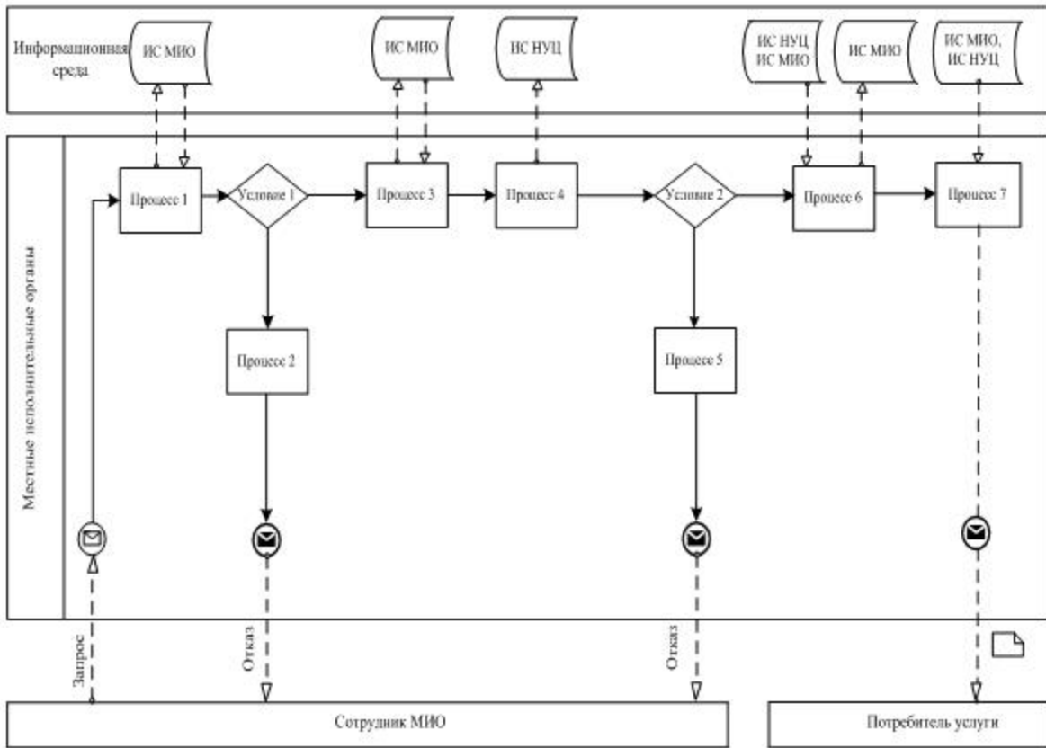
Диаграмма функционального взаимодействия при оказании «частично автоматизированной» электронной государственной услуги через ИС МЮ
