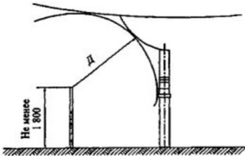
Рисунок 12. Наименьшие расстояния от контактов и ножей разъединителей в отключенном положении до заземленных и токоведущих частей
