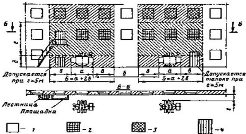
Второй вариант ( b > 4\text{ м} )
