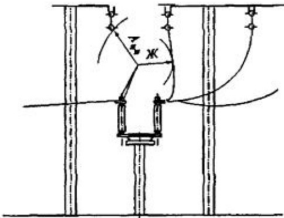
Рисунок 13. Наименьшие расстояния между токоведущими частями и зданиями и сооружениями
