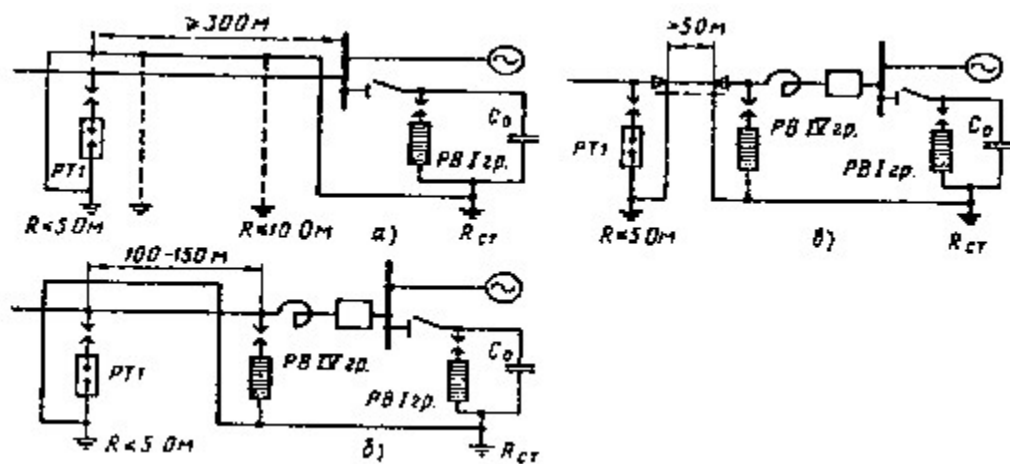
Рисунок 22. Схемы защиты электродвигателей мощностью до 3 МВт при подходе ВЛ на деревянных опорах
