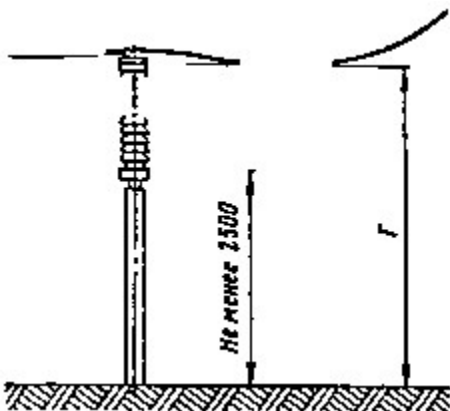
Рисунок 8. Наименьшие расстояния от токоведущих частей до транспортируемого оборудования
