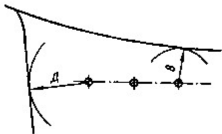
Рисунок 10. Наименьшие расстояния по горизонтали между токоведущими частями разных цепей с обслуживанием одной цепи при неотключенной другой
