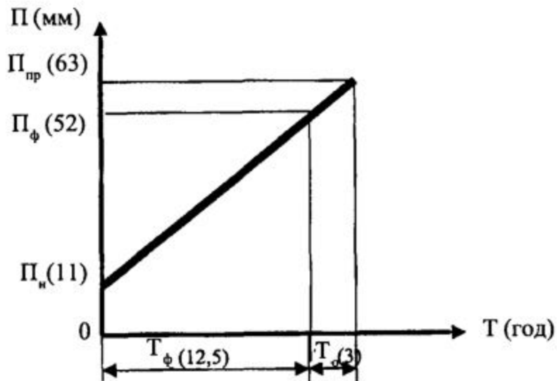
Рис. 3 Результаты расчета T_0 червячной пары
