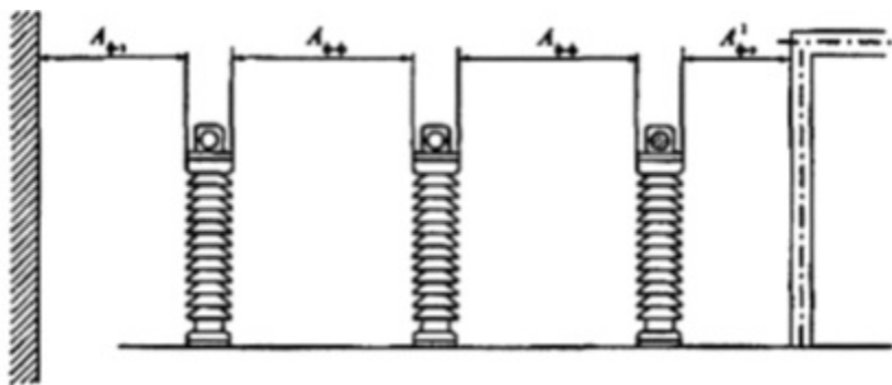
Рисунок 5. Наименьшие расстояния в свету при гибких пилах между токоведущими и заземленными частями и между токоведущими частями разных фаз, расположенными в одной горизонтальной плоскости.
