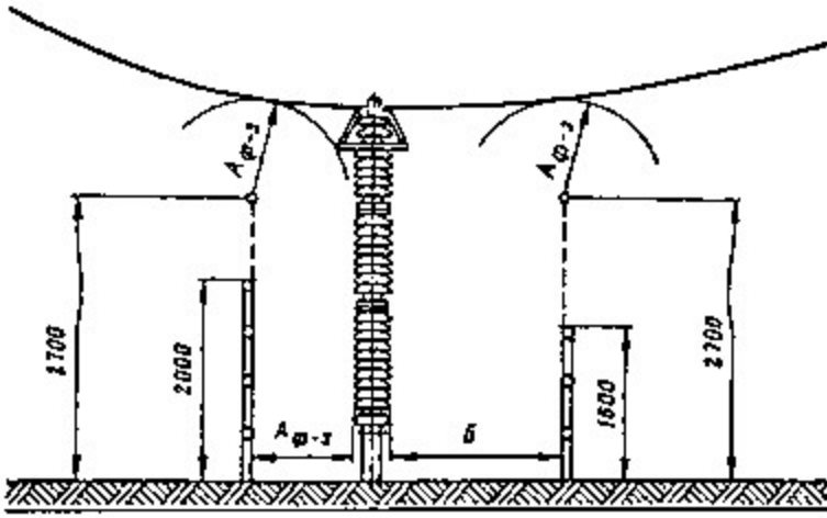
Рисунок 7. Наименьшие расстояния от неогражденных токоведущих частей и от нижней кромки фарфора изоляторов до земли
