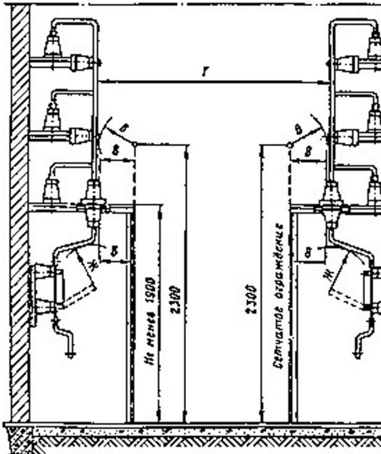
Рисунок 18. Наименьшие расстояния от пола до неогражденных неизолированных токоведущих частей и до нижней кромки фарфора изолятора и высота прохода в ЗРУ. Наименьшие расстояния от земли до неогражденных линейных выводов из ЗРУ вне территории ОРУ и при отсутствии проезда транспорта под выводами
