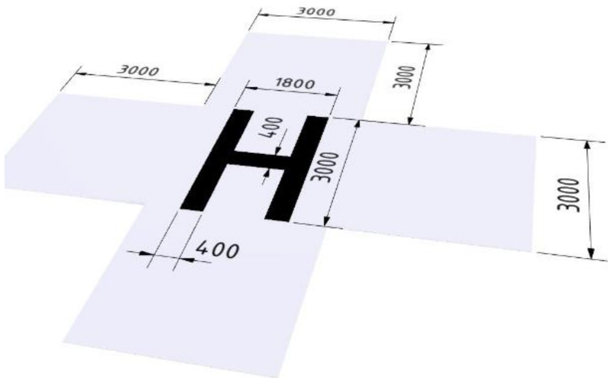
Рисунок. Оознавательная маркировка посадочной площадки при учреждении здравоохранения
